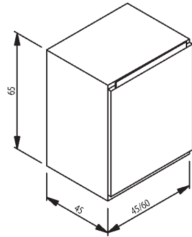
MODULO PUERTA
