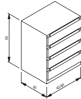
MODULO 4 CAJONES
